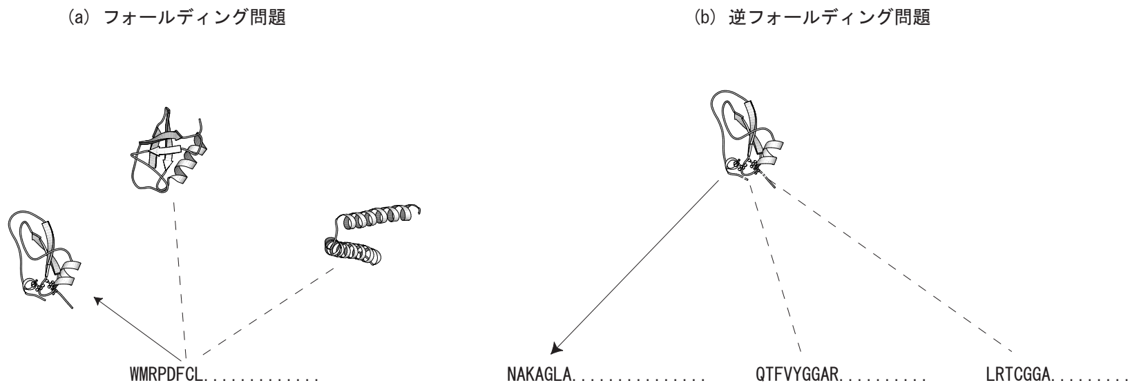
図8.11.1 フォールディング問題および逆フォールディング問題
