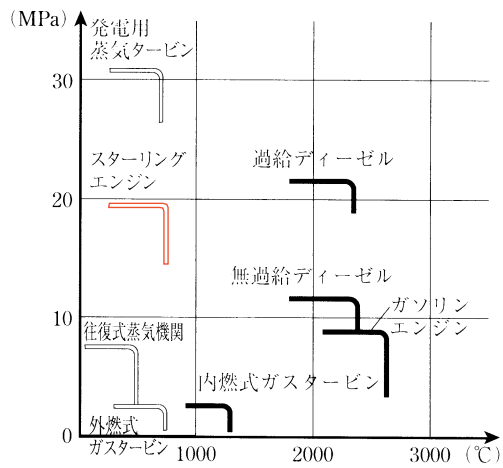
図 8.4 実機関の最高温度・最高圧力
