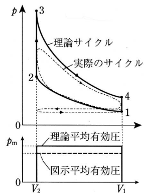
図 8.5 理論平均有効圧と図示平均有効圧
