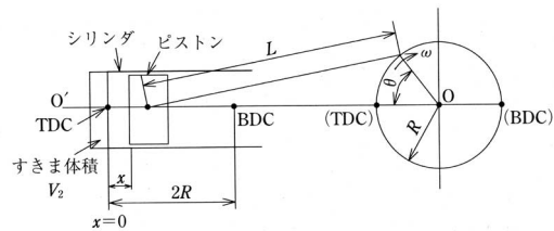
図 A ピストンクランク機構
